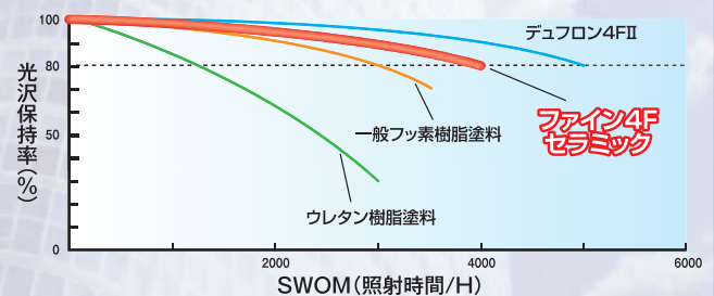
■紫外線照射(SWOM)による促進耐候性試験結果
